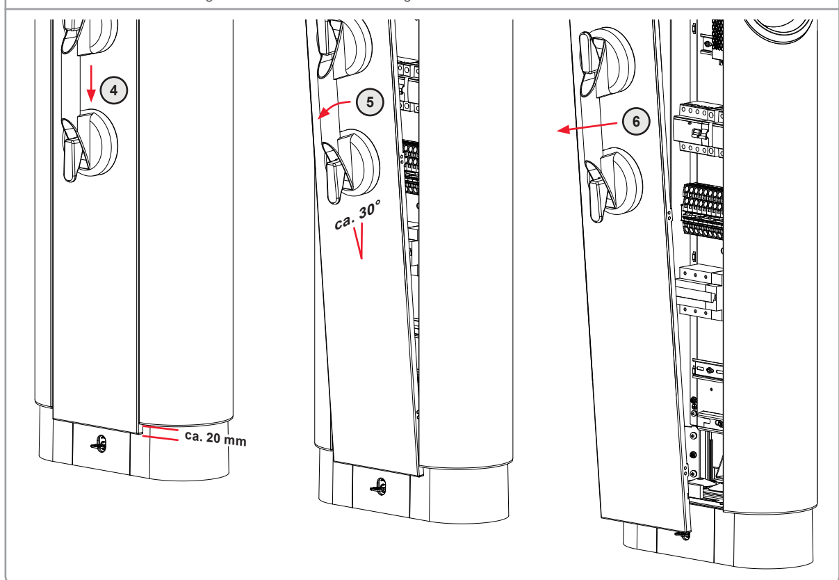
Abbildung 18: Gehäuse öffnen Technagon TEP4/TEP4 HAK – Frontblende abnehmen
