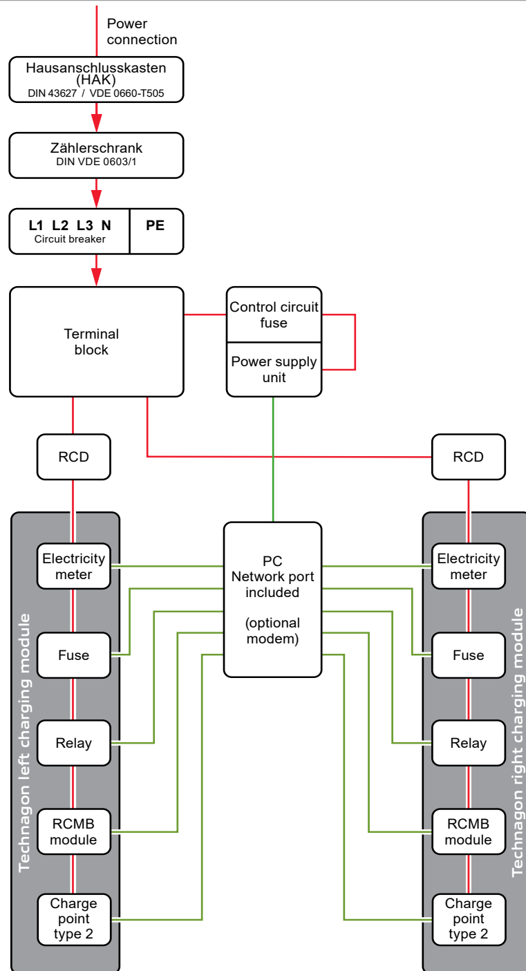
Abbildung 26: Funktionsschema Technagon TEP4 HAK
