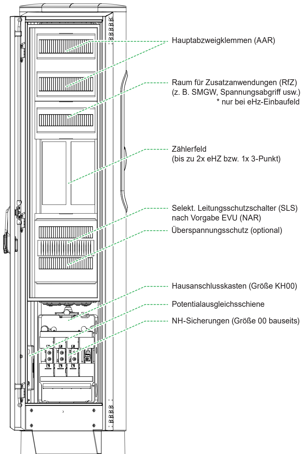
Abbildung 7: Aufbau Technagon TEP4 HAK innen
