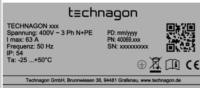
Abbildung 1: Typenschild Technagon TEP4/TEP4 HAK
