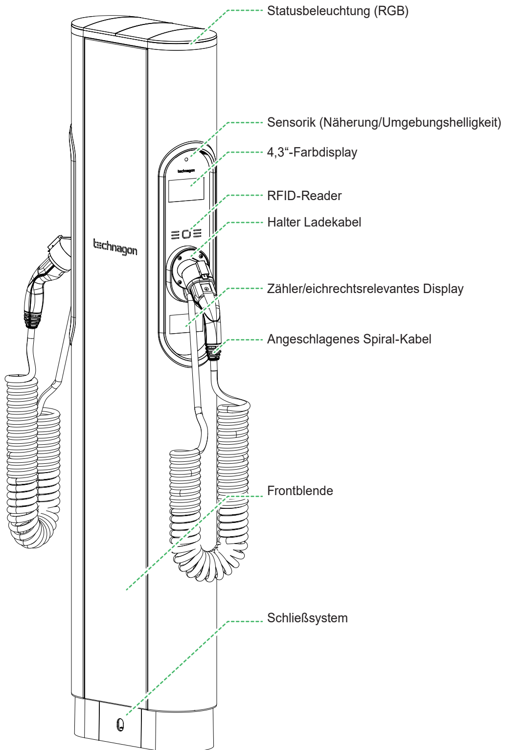
Abbildung 5: Aufbau Technagon TEP4 bei Option „angeschlagenes Spiral-Kabel“ (außen)
