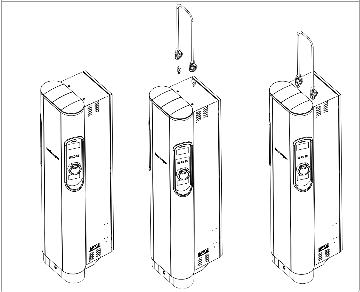
Abbildung 19: Hebevorrichtung TEP4 HAK
