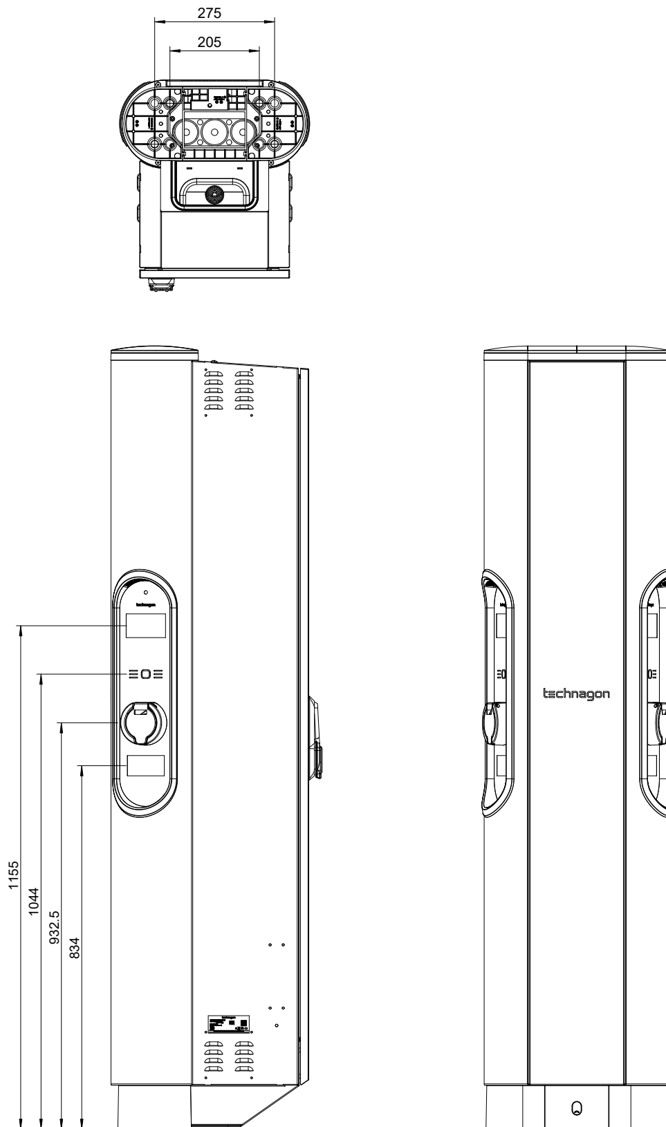
Abbildung 14: Maßübersicht Technagon TEP4 HAK - niedrige Lademodule (identische Maße siehe Abbildung 13)
