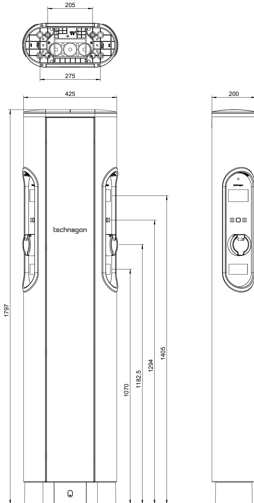
Abbildung 12: Maßübersicht Technagon TEP4
