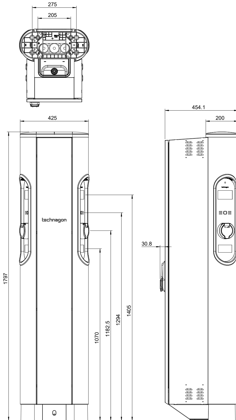
Abbildung 13: Maßübersicht Technagon TEP4 HAK
