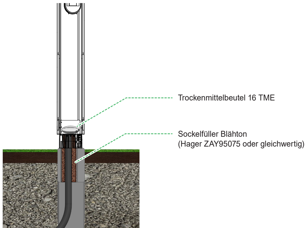
Abbildung 23: Beispiel einer Ladesäule mit ordnungsgemäßer Abdichtung und Sockelfüllmaterial
