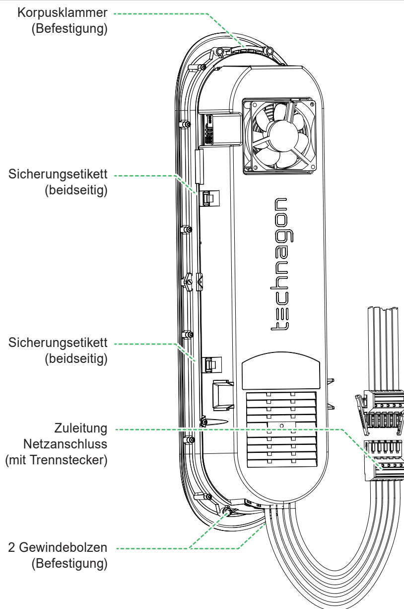
Abbildung 11: Technagon Lademodul mit zwei Gewindebolzen (de)montieren
